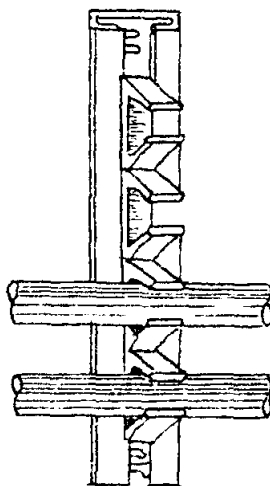
Рисунок 3 – Схема параллельной прокладки полиэтиленовых труб для электропроводки в клицах, набранных в С-образный профиль типа К-101
