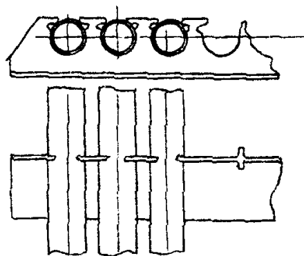
Рисунок 4 – Схема крепления полиэтиленовых труб для электропроводок в уголках из листовой стали с фасонными вырезами
